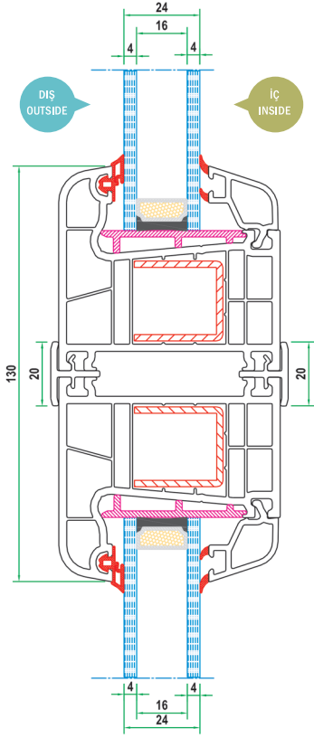
PRO 7000 KÖŞE DÖNÜŞ PROFİLİ UYGULAMASI KESİT DETAYI CORNER PIPE AND ADAPTER PROFILE SECTION DETAIL
